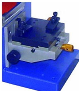
Ajuste longitudinal; transversal e em altura da mesa de impressão
