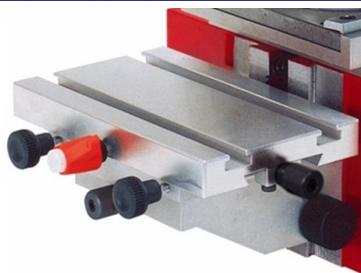
Ajuste micrométrico e altura da mesa de impressão
