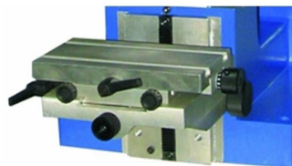
Ajuste micrométricos e de altura da mesa de colocação de peça
