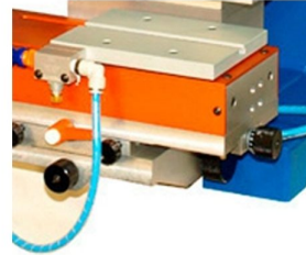
Mesa de impressão ajustável em altura e micro ajustes em eixo XX e YY
