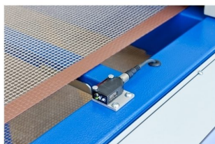
Possibilidade de equipar tunnel com fotocelula de leitura de peça para economização de energia
