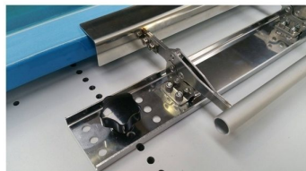
Pinça de aperto de quadro c/ aperto rápido
