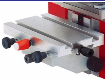
Ajuste micrométricos e altura da mesa de impressão
