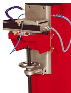
Mesa de impressão ajustável em altura através de volante; micro ajuste em eixo XX e YY
