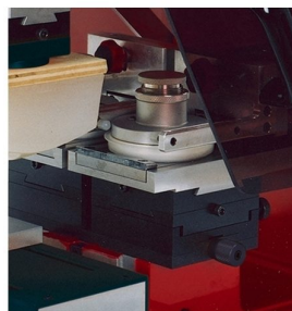
Sistema de impressão por tinteiro fechado
