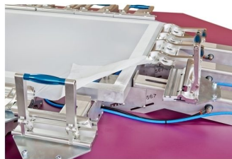
Sistema modular de acrescentimo de pinças de 200 mm
