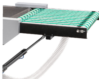
Equipado com 2x lâmpadas UV de alto rendimento "CROSS OVER" na entrada do túnel equipada com vácuo e subida/descida através de cilindros pneumáticos
