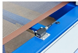
Possibilidade da colocação de cones na entrada e saída para a aspiração de fumos
