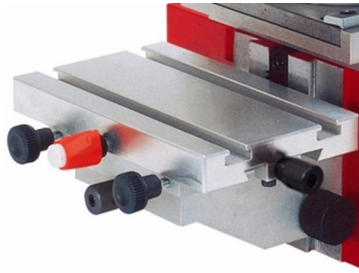
Ajuste micrométricos e altura da mesa de impressão
