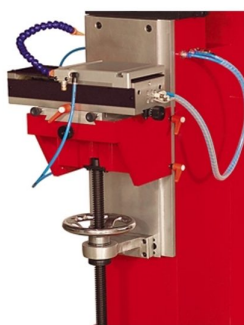
Mesa de impressão ajustável em altura através de volante; micro ajuste em eixo XX e YY
